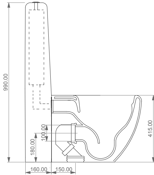
Con connessione eccentrica per scarico a suolo. ACS 102 With outlying drainage connector for floor trap. ACS 102
